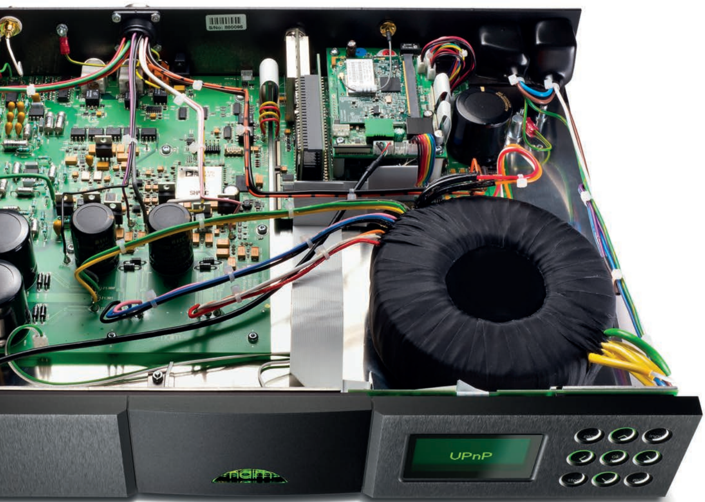
Das sorgfältig konstruierte Innenleben des Netzwerkplayers NDX mit aufwendiger Verkabelung
